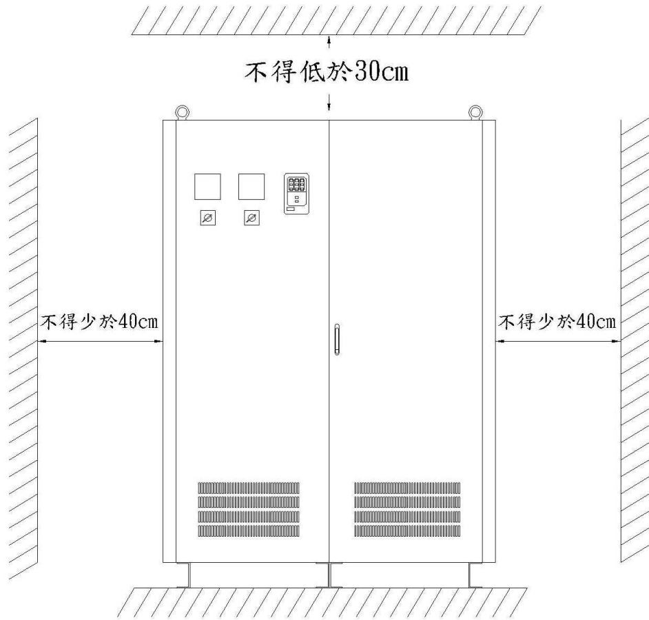
正面圖
